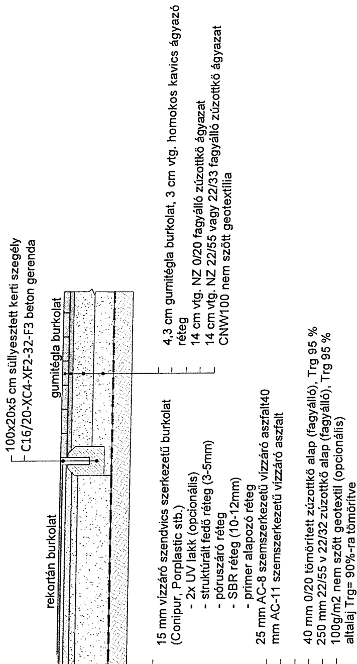
A-A metszet
