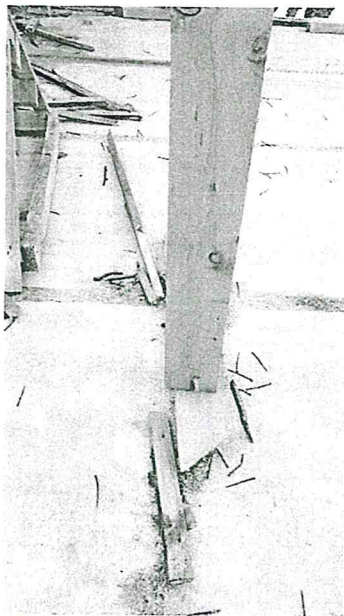
40. fénykép: Szakszerűtlen külpontos oszlop- aláékelés
