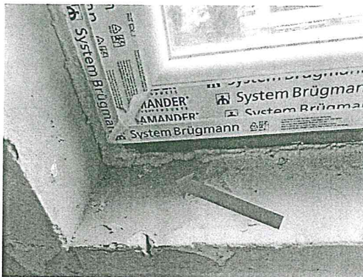
28. fénykép: A PUR-hab nem került eltakarásra
