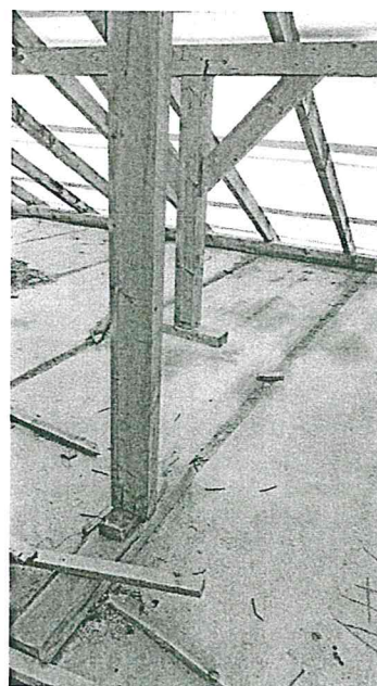
41. fénykép: Szakszerűtlen oszlop-aláékelések
