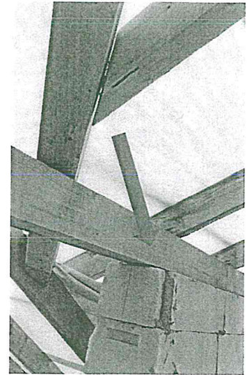
37. fénykép: Derékszelemen felfekvése
