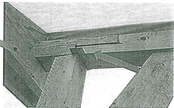
39. fénykép: Szakszerűtlen faserkezeti csomópont
