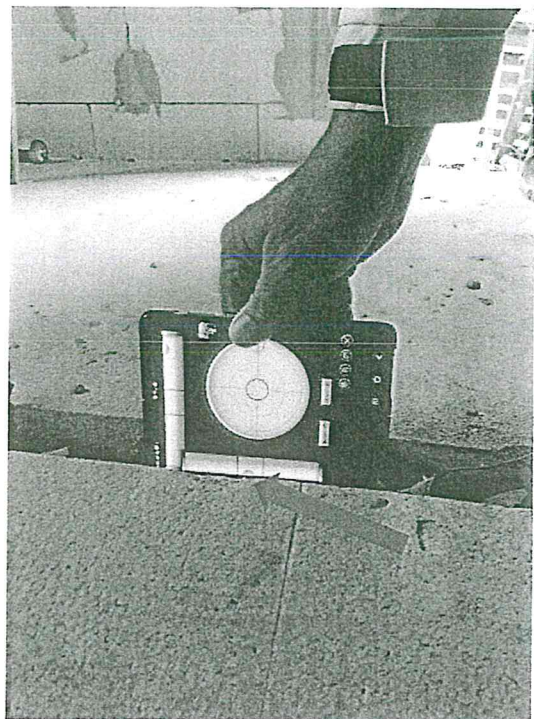
27. fénykép: A vezeték vízszintes, nem lejt.
