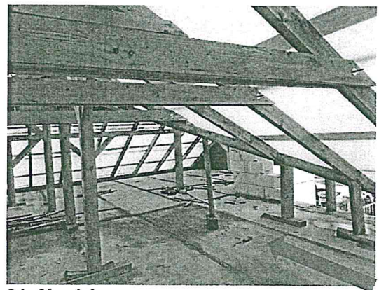
31. fénykép: A fedélszék a tervtől eltérően készült
