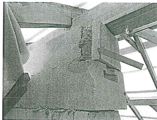
35. fénykép: Törött falazóelem „javítása” PUR-habbal
