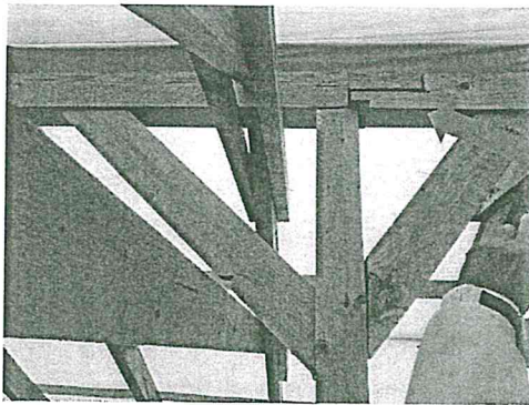
38. fénykép: Szakszerűtlen faserkezeti csomópont
